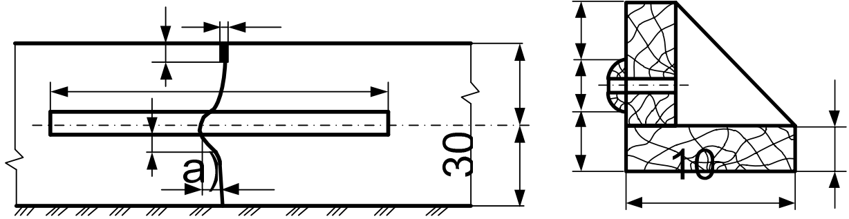
Рисунок 5.9 – Конструкція робочого шва (а) та шаблона-контурника для плити товщиною 220 мм
