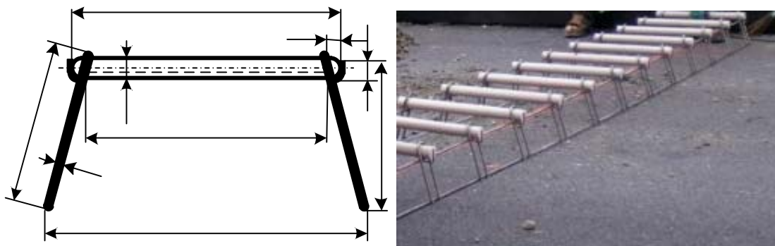
Рисунок 5.7 – Загальний вигляд та схема перерізу закладного елемента шва стискання, влаштованого за технологією розстановки закладних елементів (розміри показані в мм)
