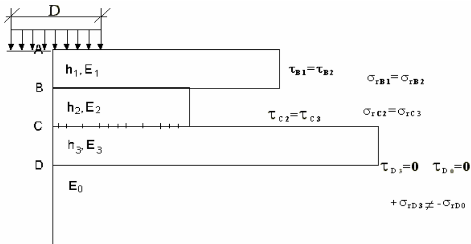
Рисунок 6.1 – Розрахункова схема дорожнього одягу з жорстким прошарком ( E_3 ). Конструкція має зчеплення покриття і жорсткого прошарку (поверхня С) та вільний контакт жорсткого прошарку і основи
