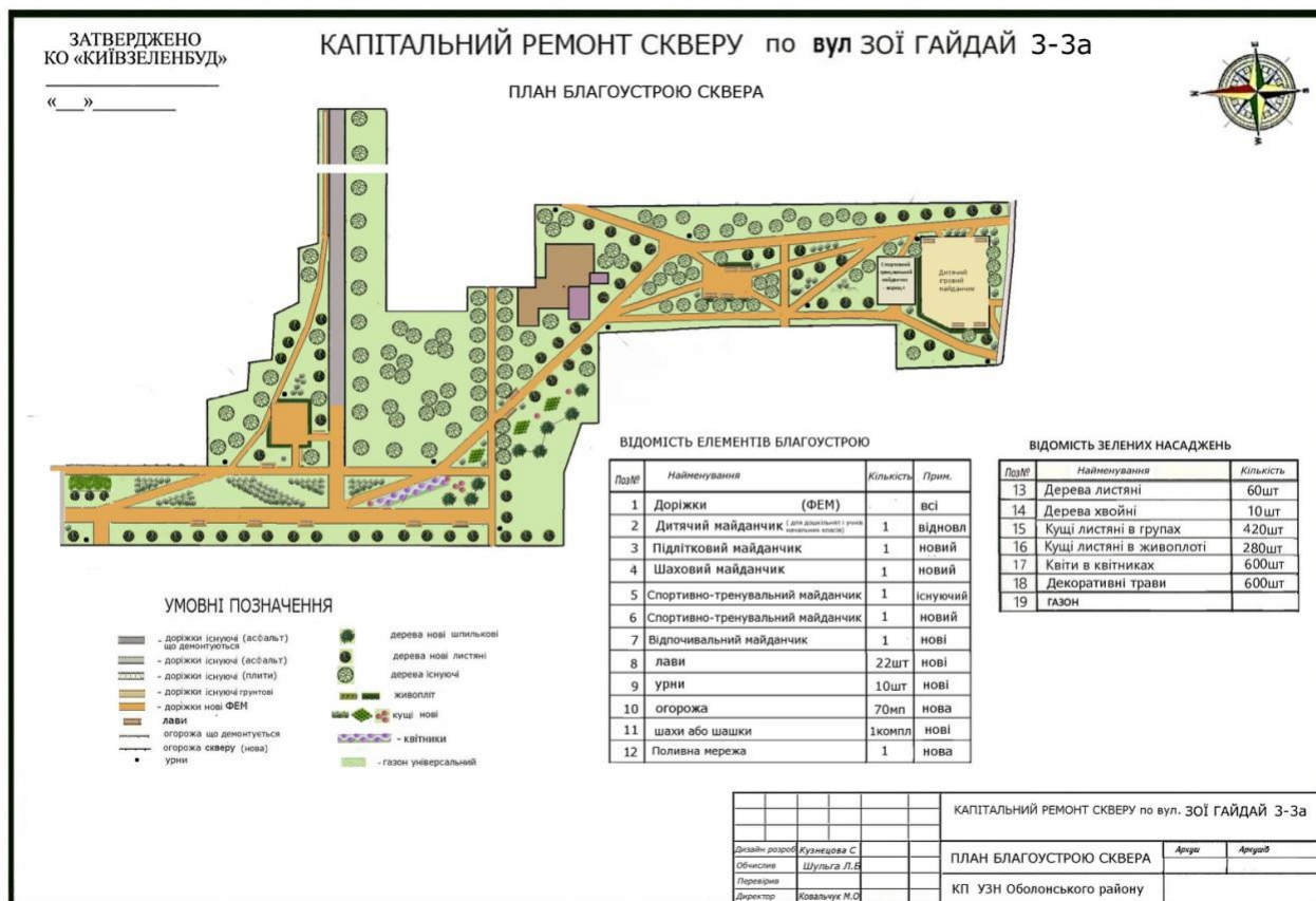
План благоустрою скверу на вул.З.Гайдай, 3-3а
