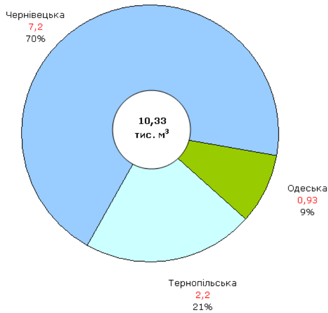
Рис. 13 - Розподіл видобутку піляльного каменю по адміністративних областях. (тис.м³)
