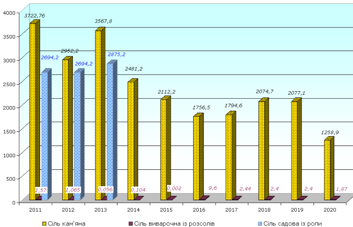
Рис. 20 - Динаміка видобутку солі кухонної за 2011-2020 рр. (тис.т)
