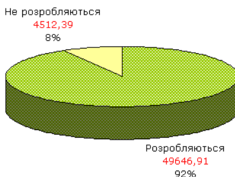
Рис. 17 - Розподіл балансових запасів польовошпатової сировини за ступенем промислового освоєння
