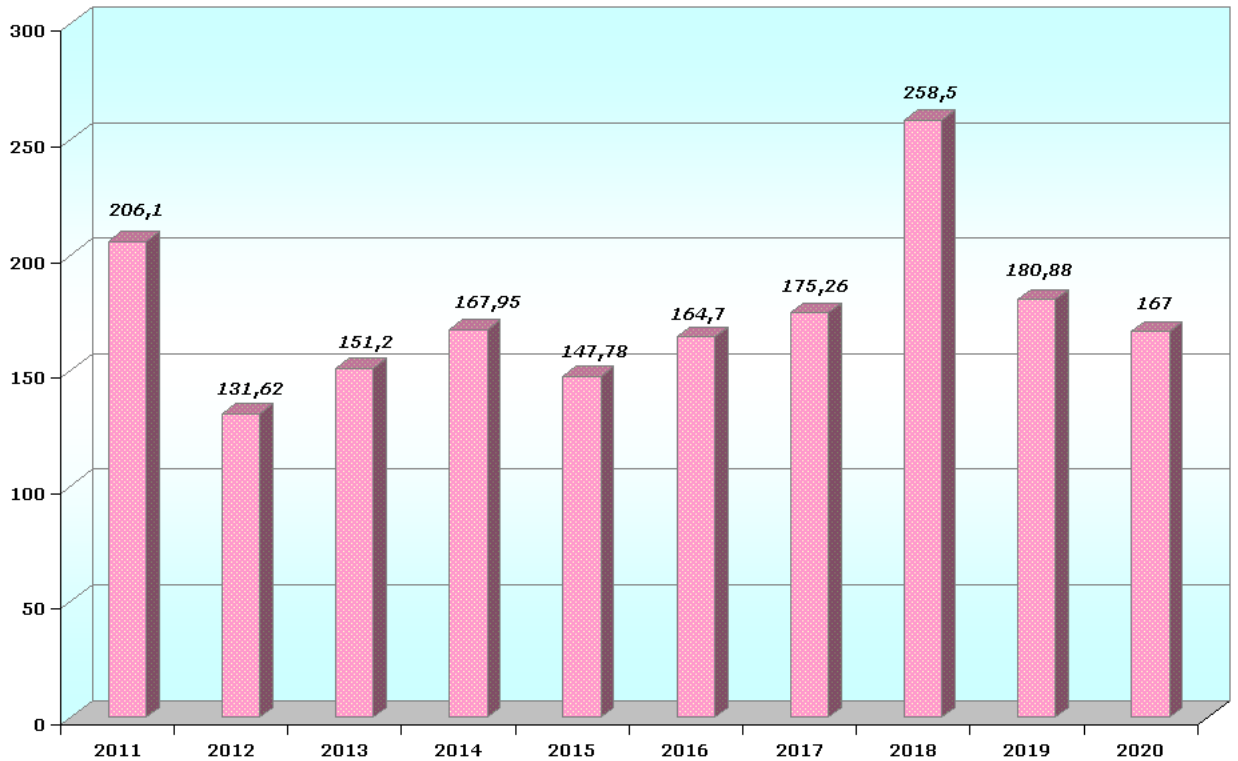
Рис. 27 - Динаміка видобутку сировини для мінеральної вати та волокон за 2011-2020 рр. (тис.т)
