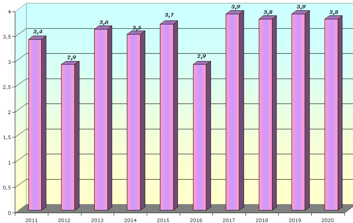
Рис. 8 - Динаміка видобутку марганцевих руд (млн.т) за 2011-2020 рр.
