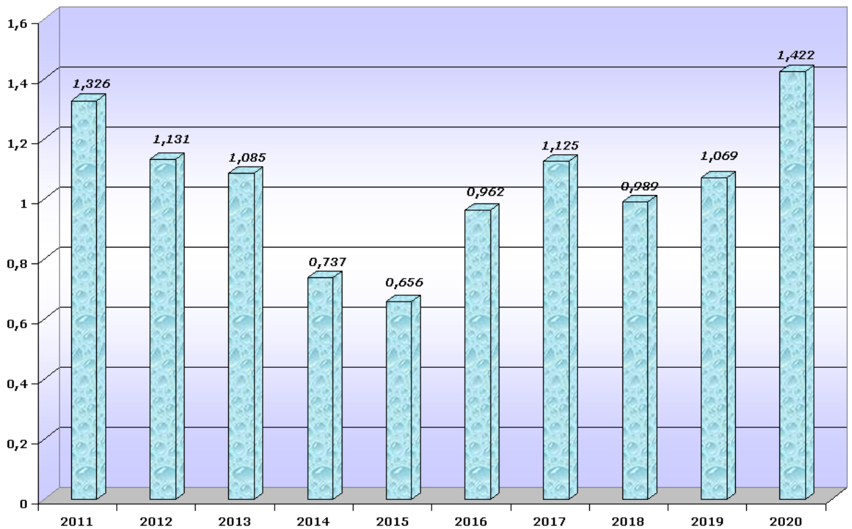
Рис. 25 - Динаміка видобутку скляної сировини за 2011-2020 рр., (млн.т)
