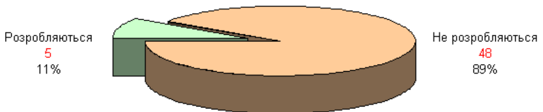
Рис. 35 - Розподіл родовищ за ступенем промислового освоєння (кількість родовищ)
