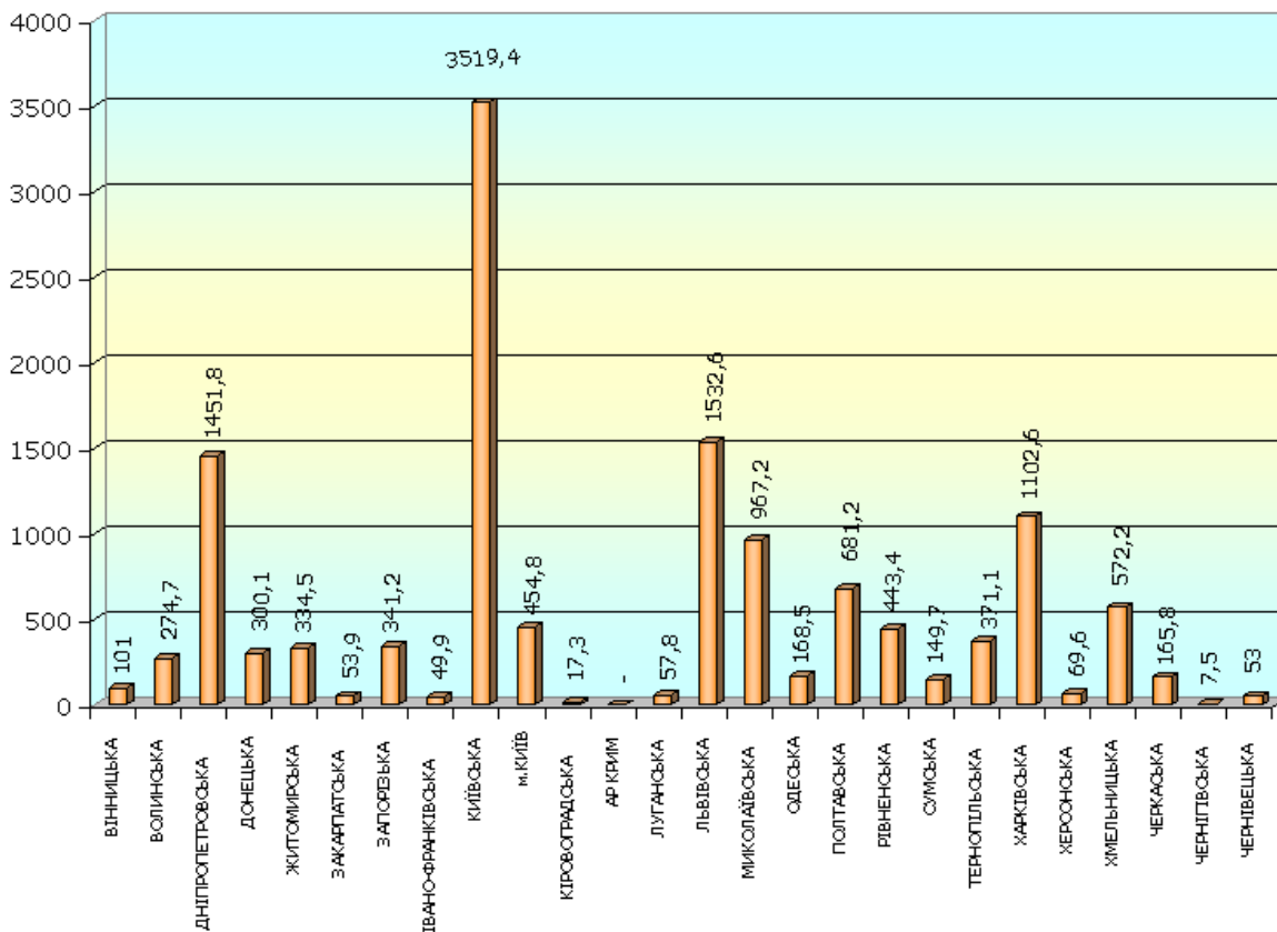
Рис. 21 - Видобуток у 2020 році піску будівельного по адміністративних областях (тис. м³)
