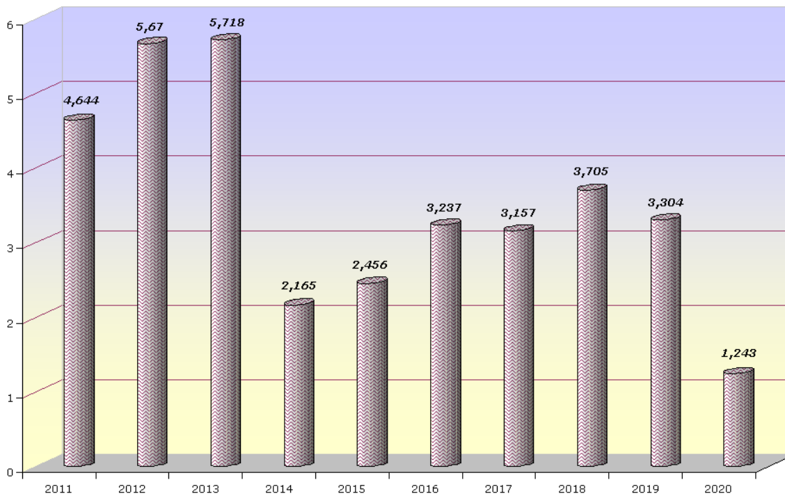
Рис. 10 - Динаміка видобутку лікувальних грязей за 2011-2020 рр.(тис.м³)
