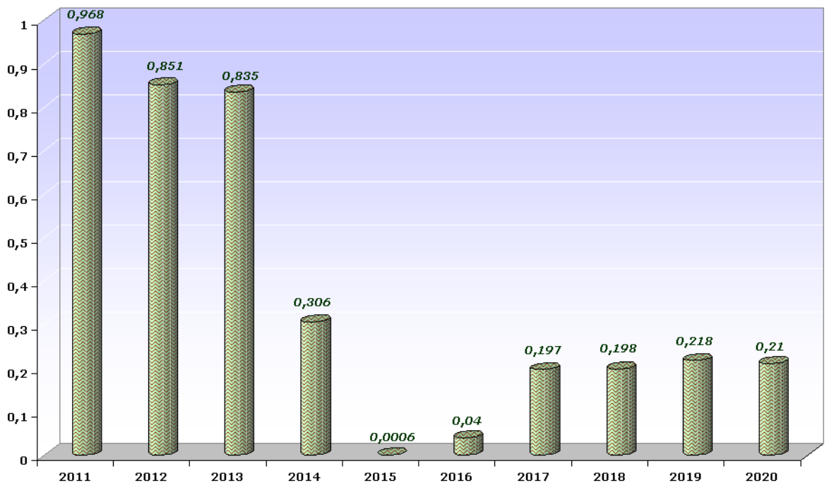
Рис. 2 - Динаміка видобутку тугоплавких глин за 2011-2020 рр., (млн.т)
