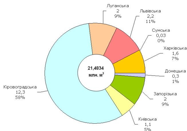
Рис. 24 - Розподіл балансових запасів сировини для закладання виїмкового простору по адміністративних областях (млн.м³)
