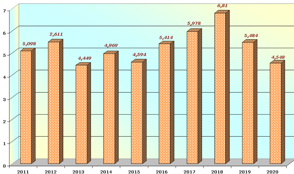
Рис. 3 - Динаміка видобутку вогнетривких глин за 2011-2020 рр., (млн.т)
