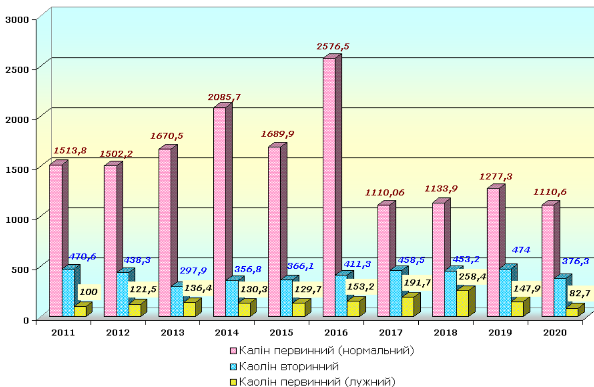
Рис. 7 - Динаміка видобутку каоліну за 2011-2020 рр., (тис.т)
