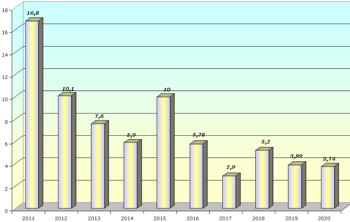
Рис. 41 - Динаміка видобутку перлітової сировини за 2011-2020 рр., (тис.м³)
