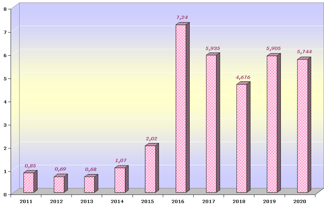
Рис. 31 - Динаміка видобутку сировини карбонатної для виробництва вапна за 2011-2020 рр. (млн.т)
