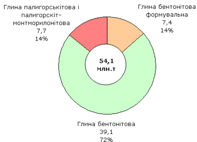
Рис. 3 - Розподіл балансових запасів бентонітових глин за видами, (млн.т)
