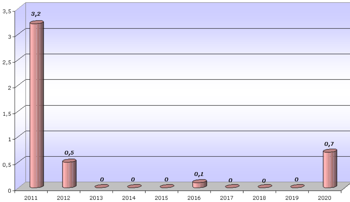
Рис. 37 - Динаміка видобутку крем'яної сировини за 2011-2020 рр., (тис.т)
