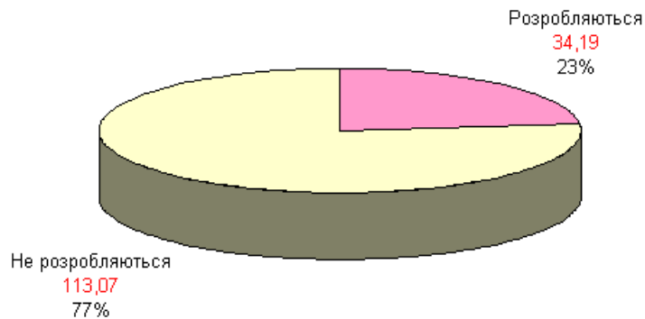
Рис. 28 - Розподіл балансових запасів за ступенем промислового освоєння (млн. т)
