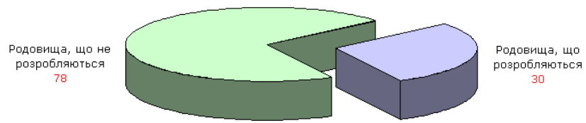
Рис. 29 - Розподіл балансових запасів за ступенем промислового освоєння (кількість родовищ)
