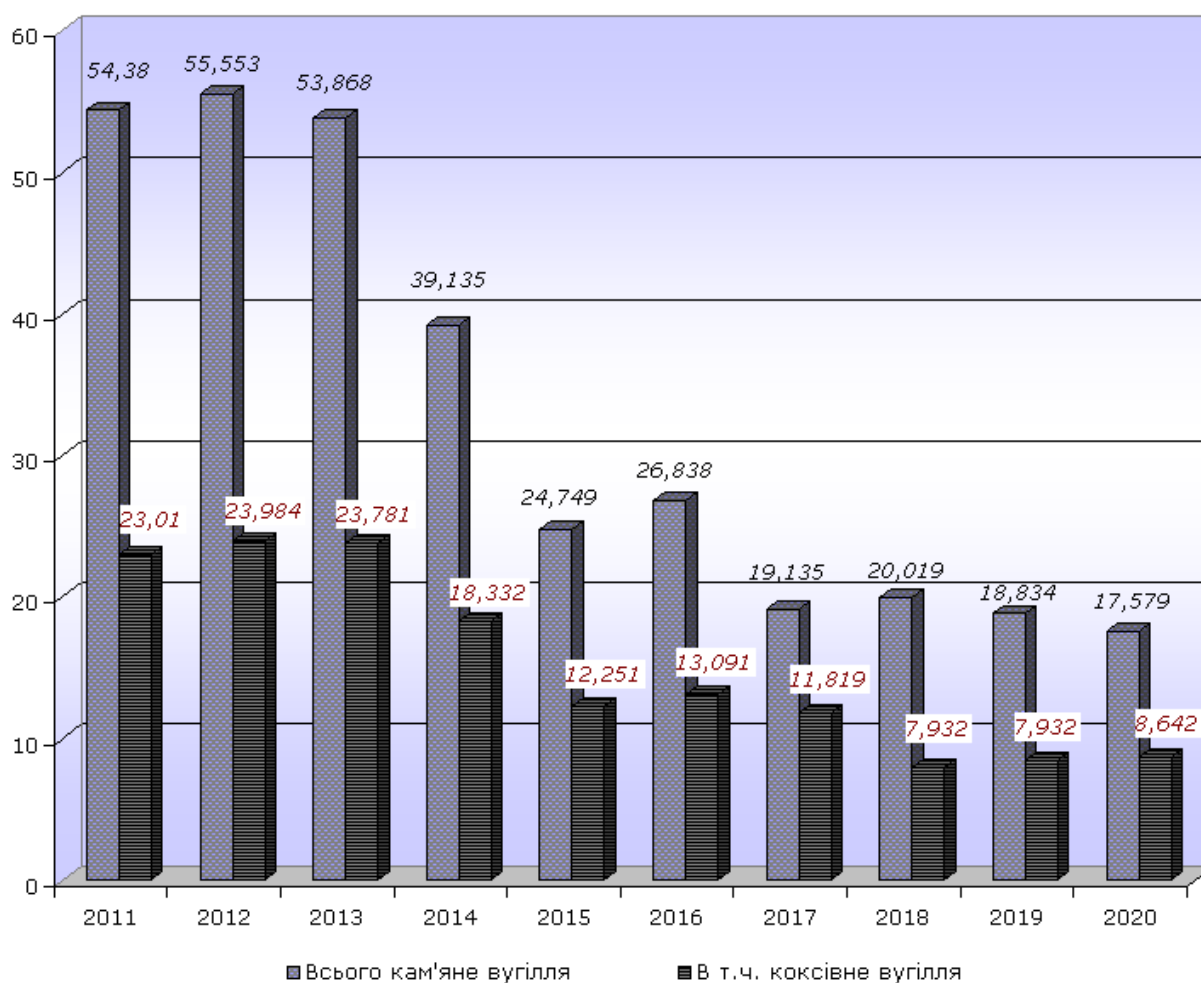
Рис. 3 - Динаміка видобутку кам'яного вугілля в Україні за 2011-2020 роки, (млн.т)
