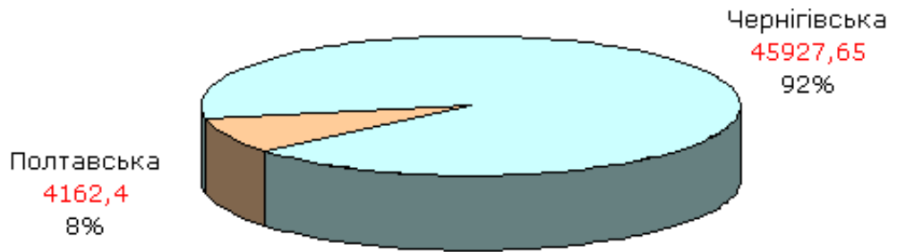
Рис. 3 - Розподіл балансових запасів бішофіту по адміністративних областях (тис. т)
