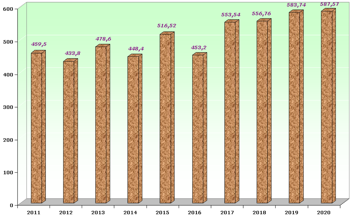
Рис. 6 - Динаміка видобутку каменю облицювального за 2011-2020 рр., (тис.м³)
