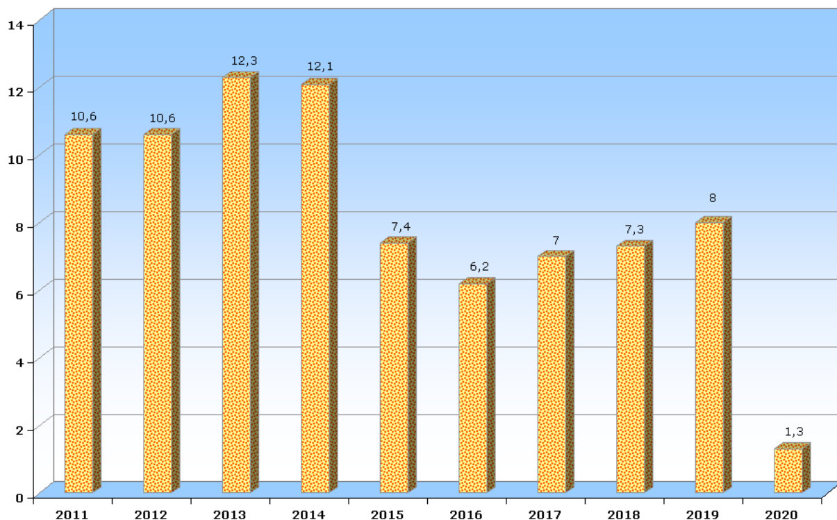
Рис. 12 - Динаміка видобутку пісків формувальних в Україні (млн.т).
