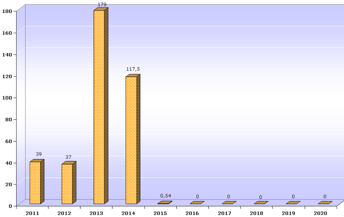
Рис. 22 - Динаміка видобутку сировини за 2011-2020 рр., (тис.м³)
