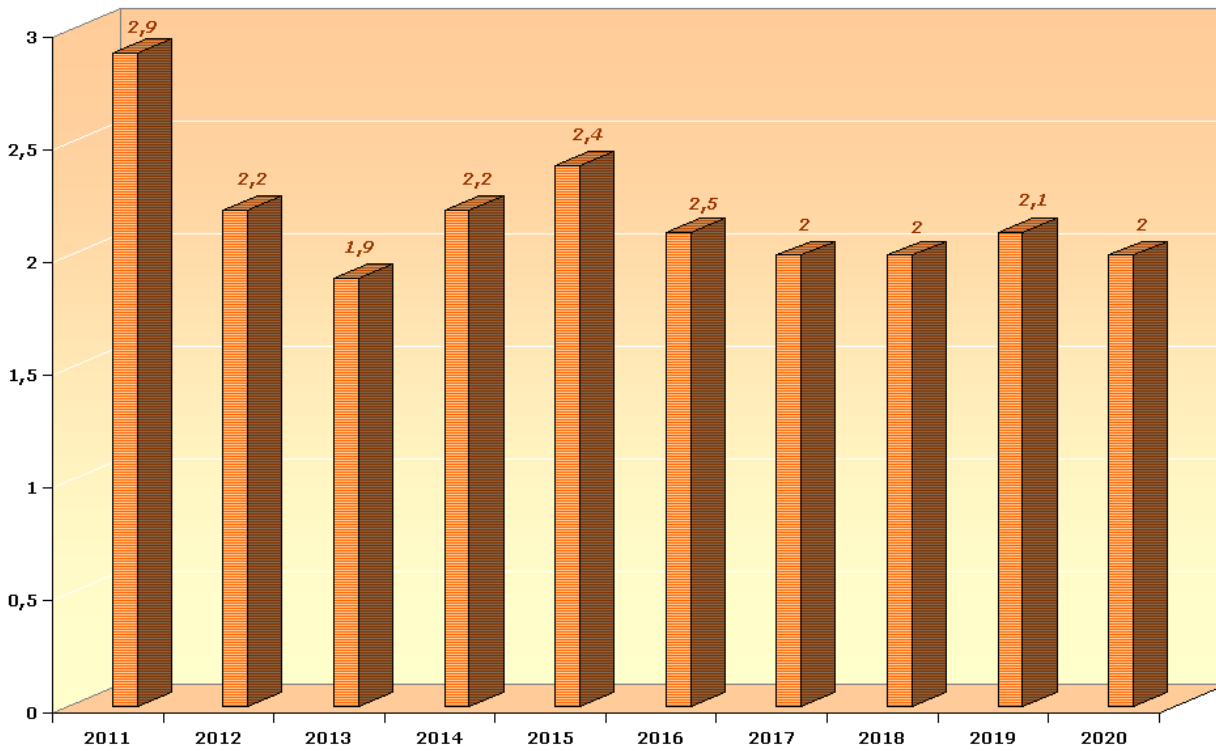
Рис. 44 - Динаміка видобутку цегельно-черепичної сировини за 2011-2020 рр., (млн.м³)
