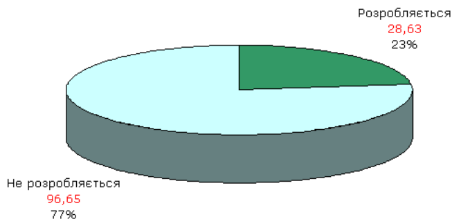
Рис. 21 - Розподіл балансових запасів цеолітової сировини за ступенем промислового освоєння родовищ (млн. т)
