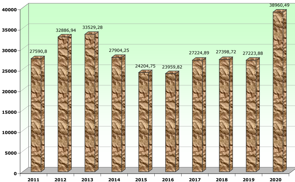
Рис. 4 - Динаміка видобутку каменю будівельного за 2011-2020 рр.,(тис.м 3 )
