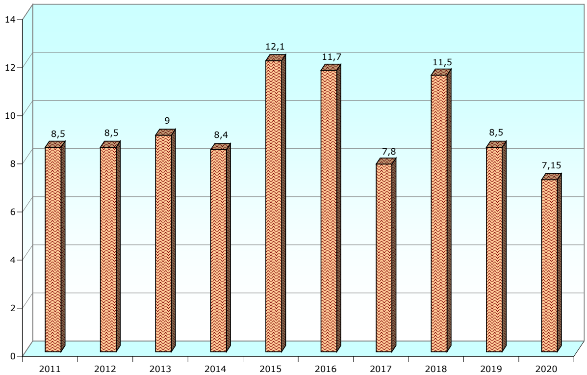
Рис. 4 - Динаміка видобутку бішофіту за 2011-2020 рр. (тис.т)
