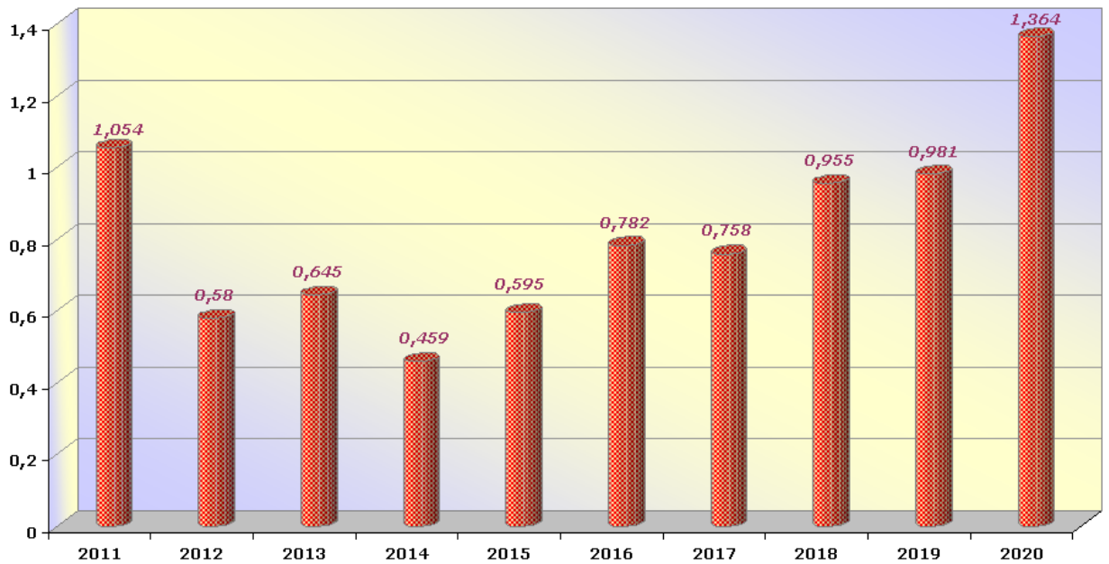
Рис. 6 - Динаміка видобутку доломіту для металургії за 2011-2020 рр., (млн.т)
