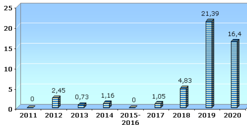
Рис. 50 - Динаміка видобутку менілітових сланців за 2011-2020 рр., (тис.т)
