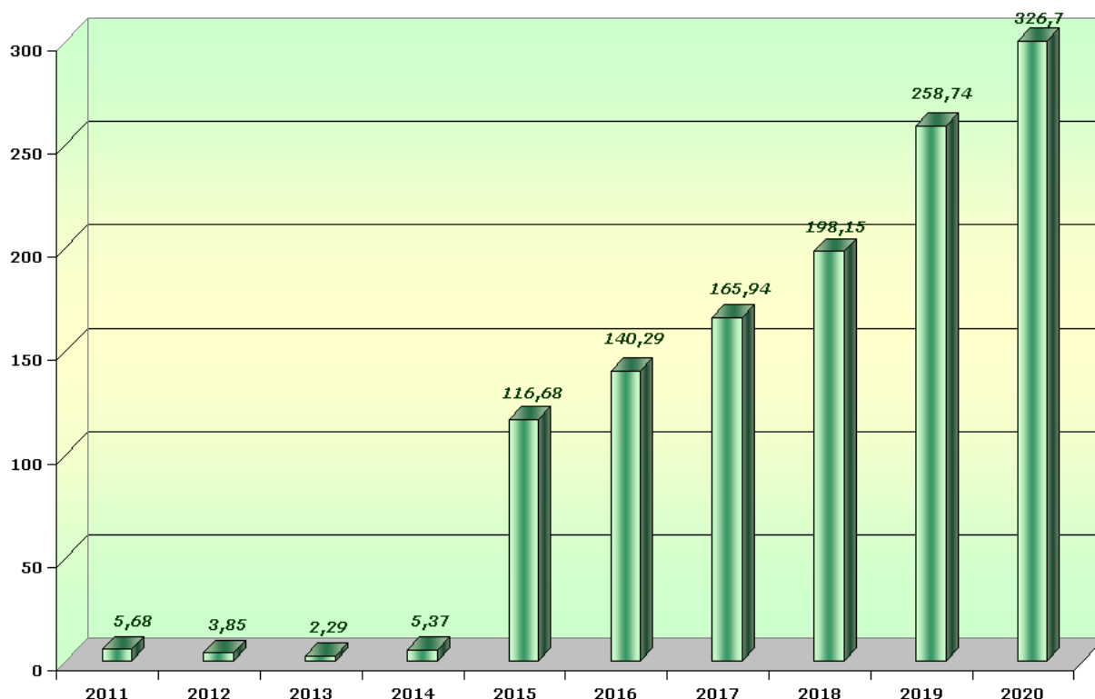
Рис. 20 - Динаміка видобутку цеолітової сировини за 2011-2020 рр., (тис. т)
