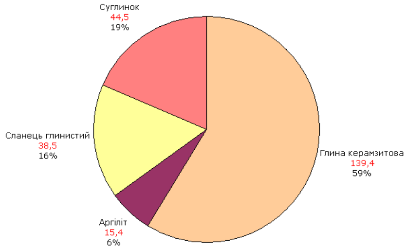
Рис. 33 - Розподіл балансових запасів керамзитової сировини за видами порід, (млн. м³)
