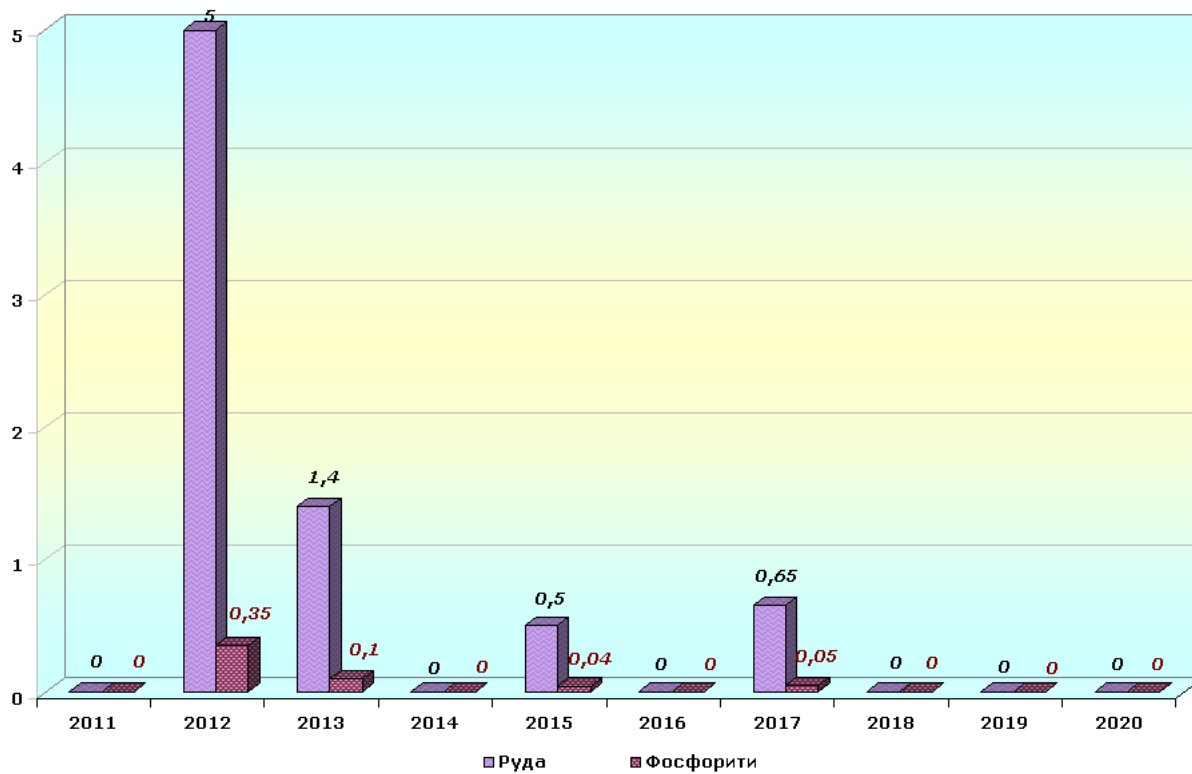
Рис. 24 - Динаміка видобутку фосфоритів в 2011-2020 рр (млн.т)
