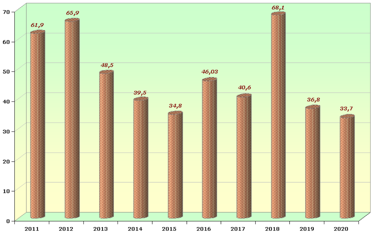
Рис. 34 - Динаміка видобутку керамзитової сировини за 2011-2020 рр., (тис.м³)
