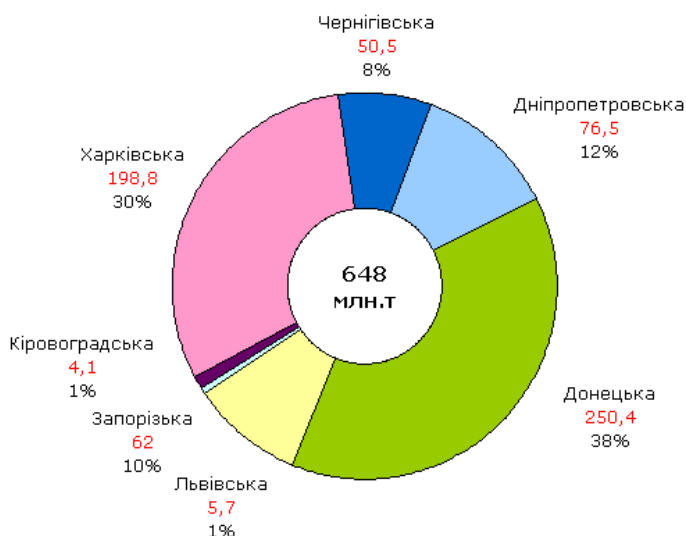
Рис. 11 - Розподіл балансових запасів піску формувального по адміністративних областях, (млн.т)
