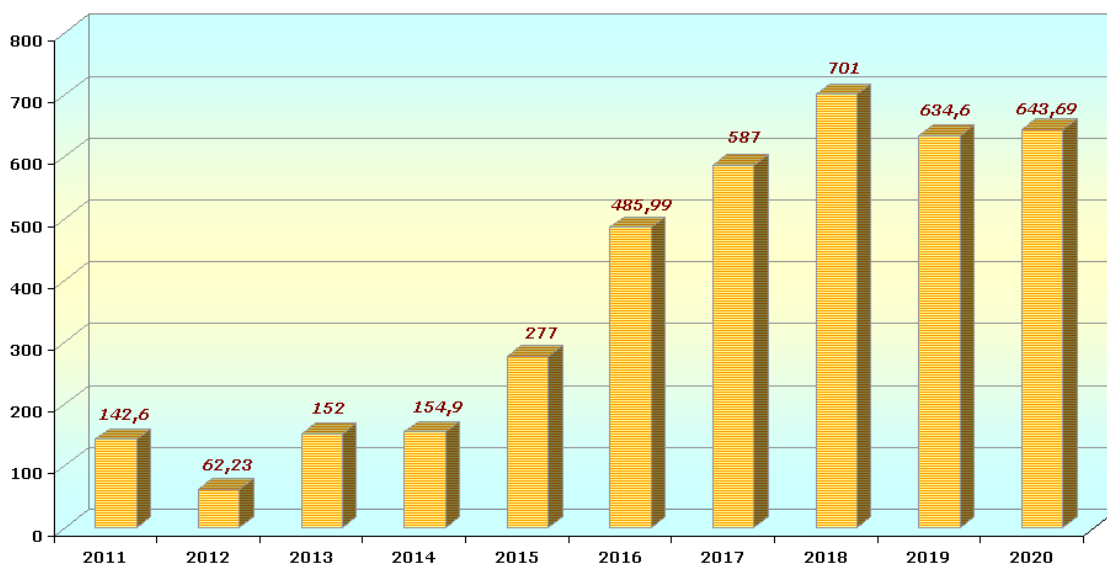
Рис. 14 - Динаміка видобутку польовошпатової сировини за 2011-2020 рр. (тис.т)
