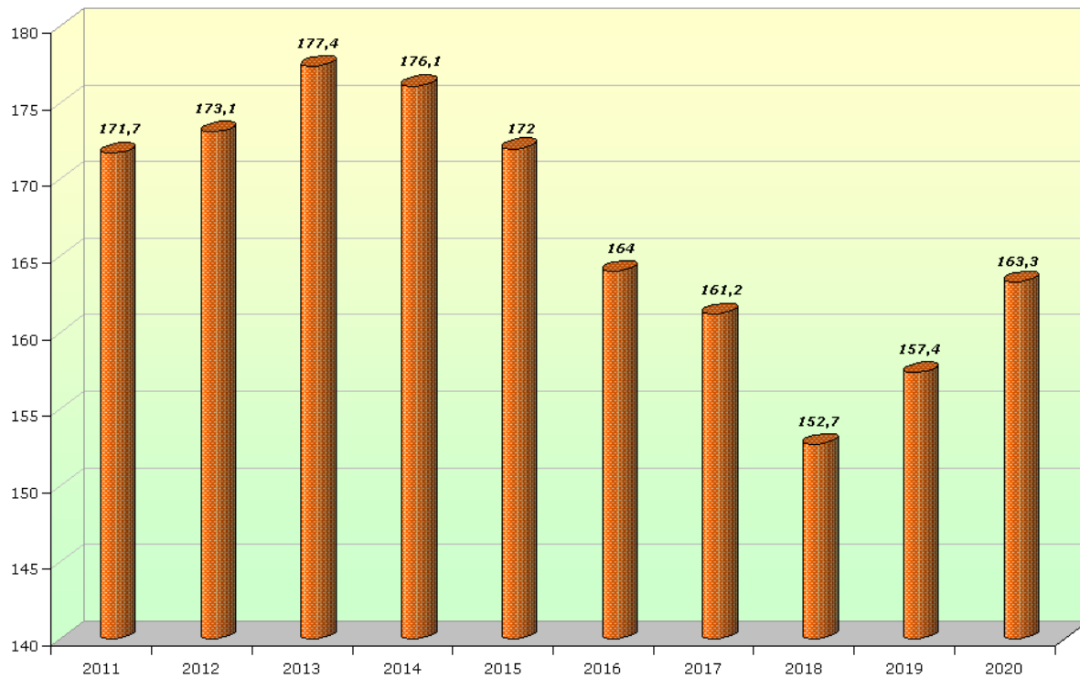
Рис. 4 - Динаміка видобутку залізних руд за 2011-2020 рр. (млн.т)
