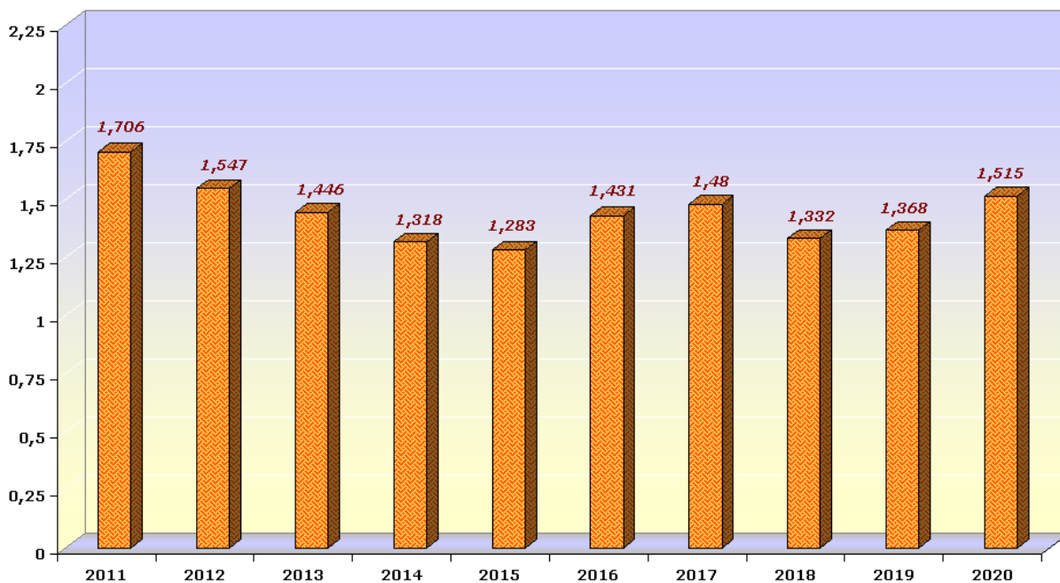
Рис. 1 - Динаміка видобутку гіпсу та ангідриту в Україні за 2011-2020 рр., (млн.т)
