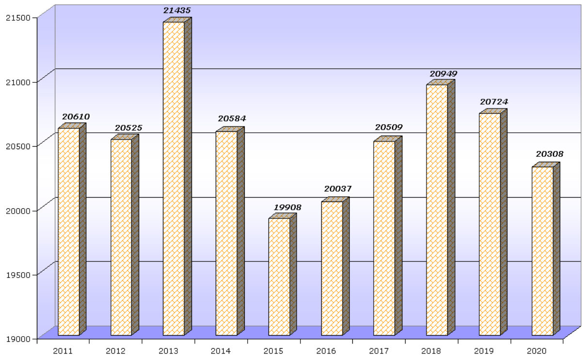
Рис. 2 - Динаміка видобутку природного газу за 2011-2020 рр., (млн.м³)
