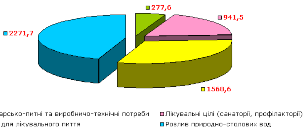
Рис. 5 - Використання підземних мінеральних вод по Україні (м³/добу)
