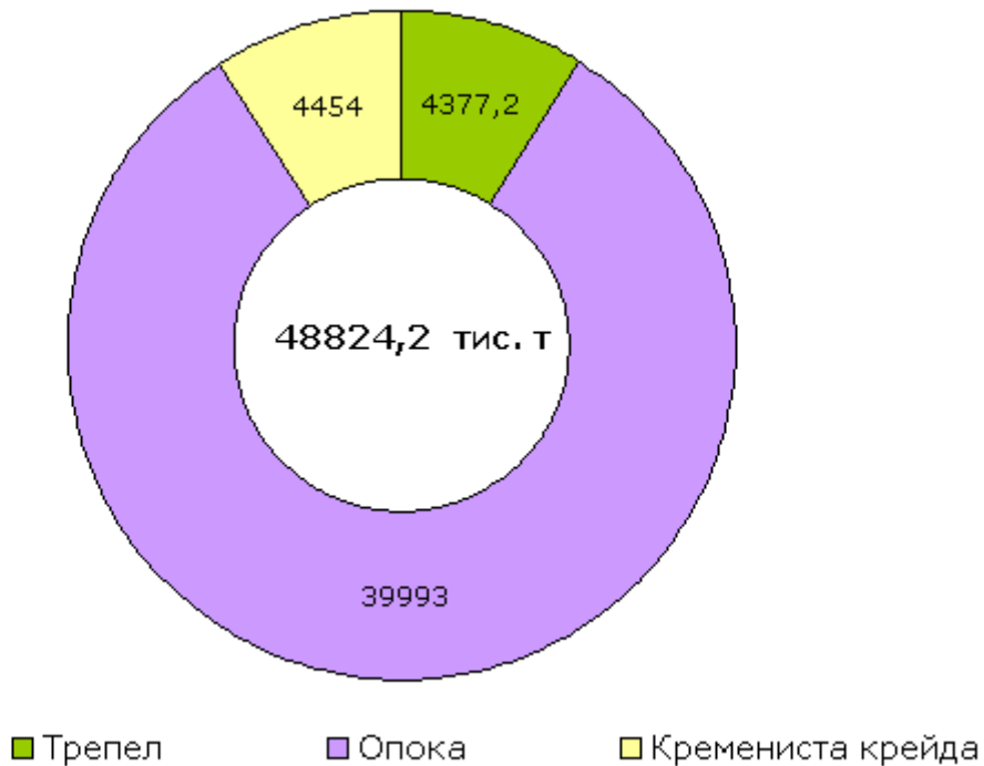
Рис. 38 - Розподіл балансових запасів за видами сировини, (тис.т)
