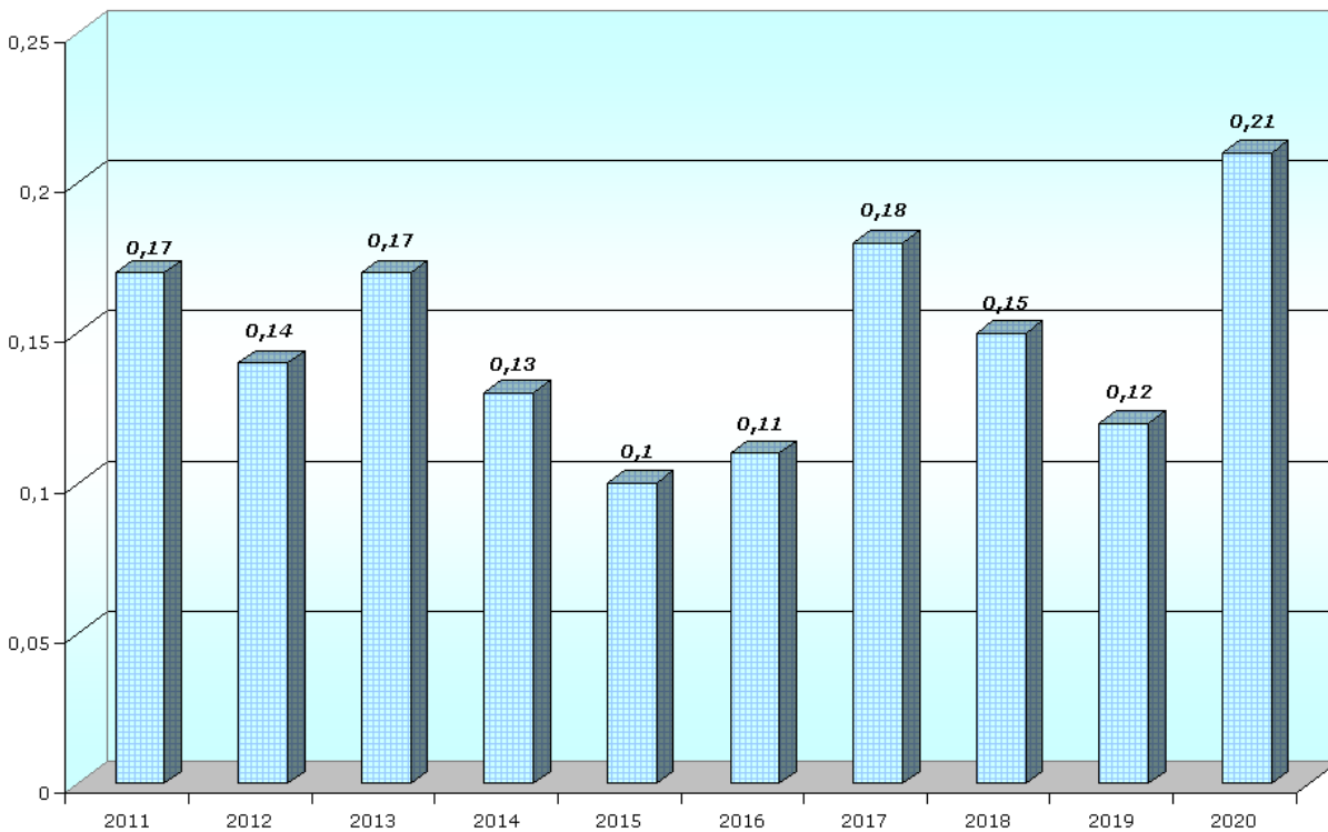
Рис. 19 - Динаміка видобутку крейди за 2011-2020 рр., (млн.т)
