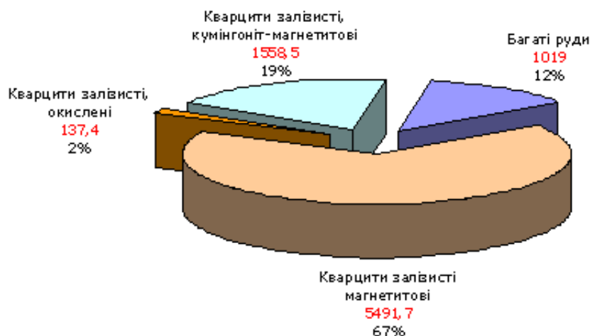
Рис. 1 - Розподіл запасів родовищ, що перебувають в розробці, за типами руд за 2020 р. (за кат.А+В+С 1 , млн.т)
