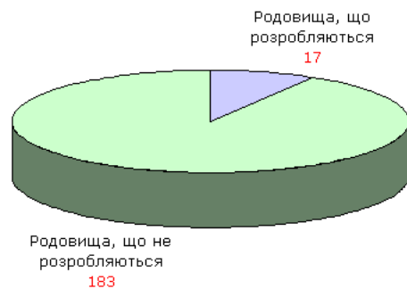
Рис. 14 - Розподіл балансових запасів за ступенем промислового освоєння (кількість родовищ)
