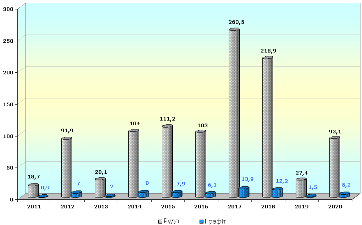
Рис. 4 - Динаміка видобутку руд графітових за 2011-2020 рр. (тис.т)
