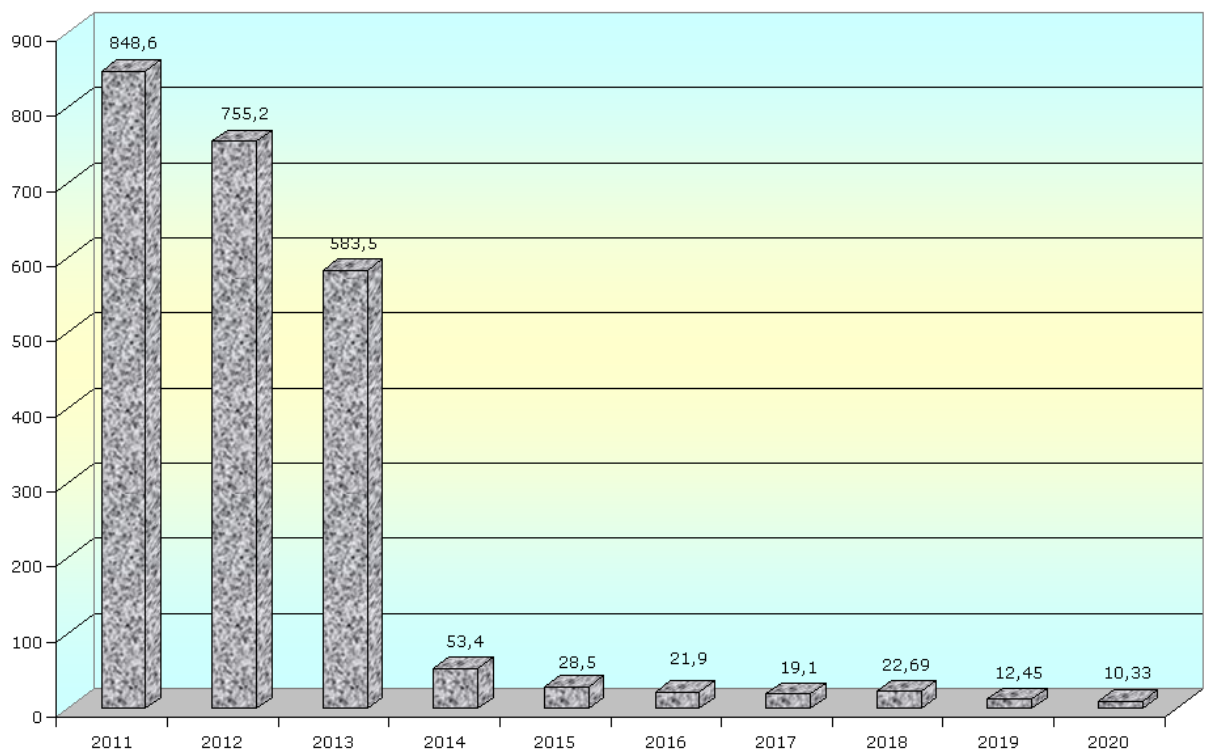
Рис. 16 - Динаміка видобутку пиляльних вапняків за 2011-2020р., (тис.м³).
