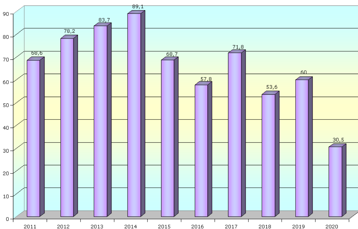
Рис. 16 - Динаміка видобутку ставроліту за 2011-2020 рр.,(тис.т)
