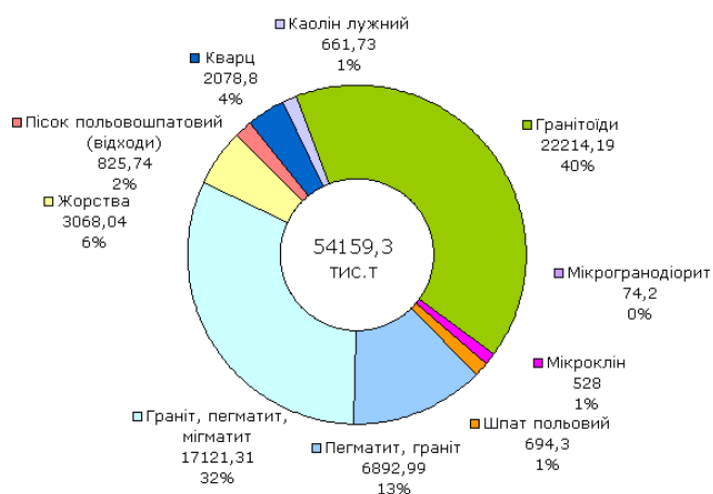
Рис. 16 - Розподіл балансових запасів польовошпатової сировини за типами (тис.т)
