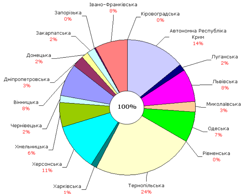
Рис. 30 - Розподіл запасів родовищ вапняку для випалювання на вапно по адміністративних областях, (%)
