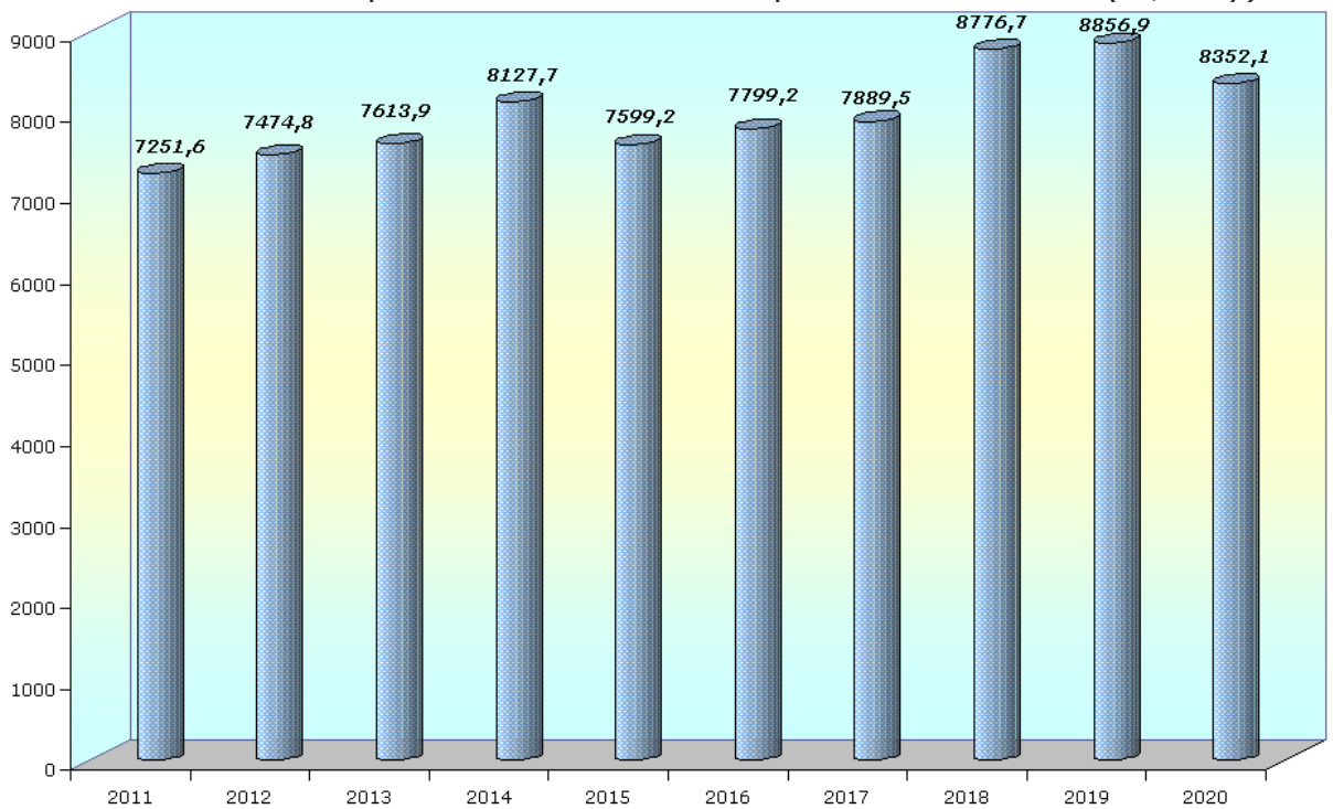
Рис. 3 - Динаміка видобутку підземних мінеральних вод за 2011-2020 рр. (м³/добу)
