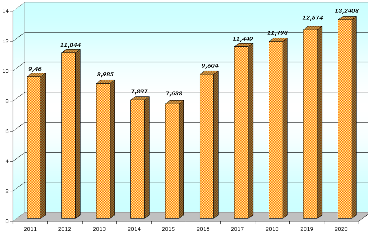
Рис. 20 - Динаміка видобутку піску будівельного за 2011-2020 рр. (млн.м³)
