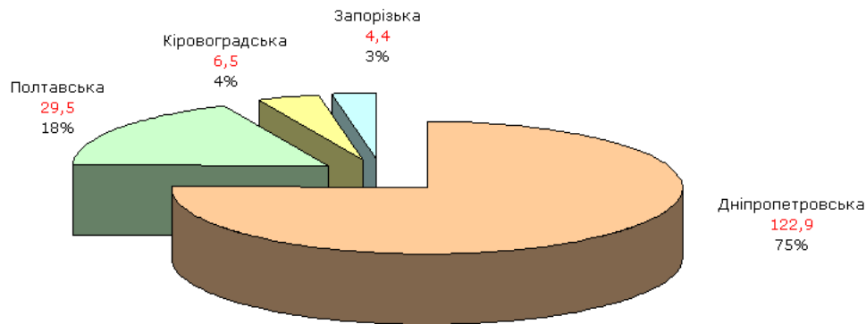
Рис. 5 - Розподіл видобутку залізних руд по адміністративних областях (млн.т)
