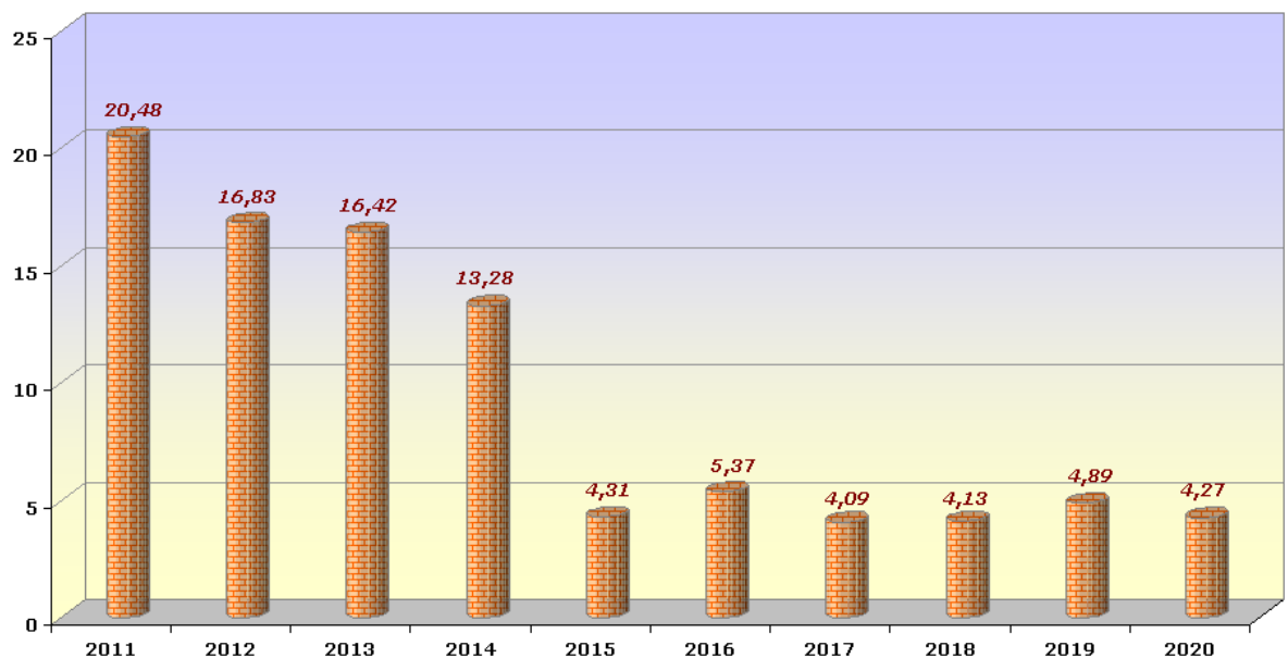
Рис. 2 - Динаміка видобутку флюсової сировини за 2011-2020 рр., (млн.т)
