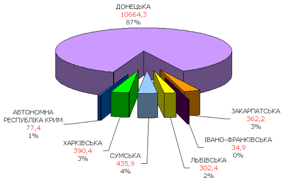
Рис. 22 - Розподіл балансових запасів солі кухонної по адміністративних областях (млн.т)
