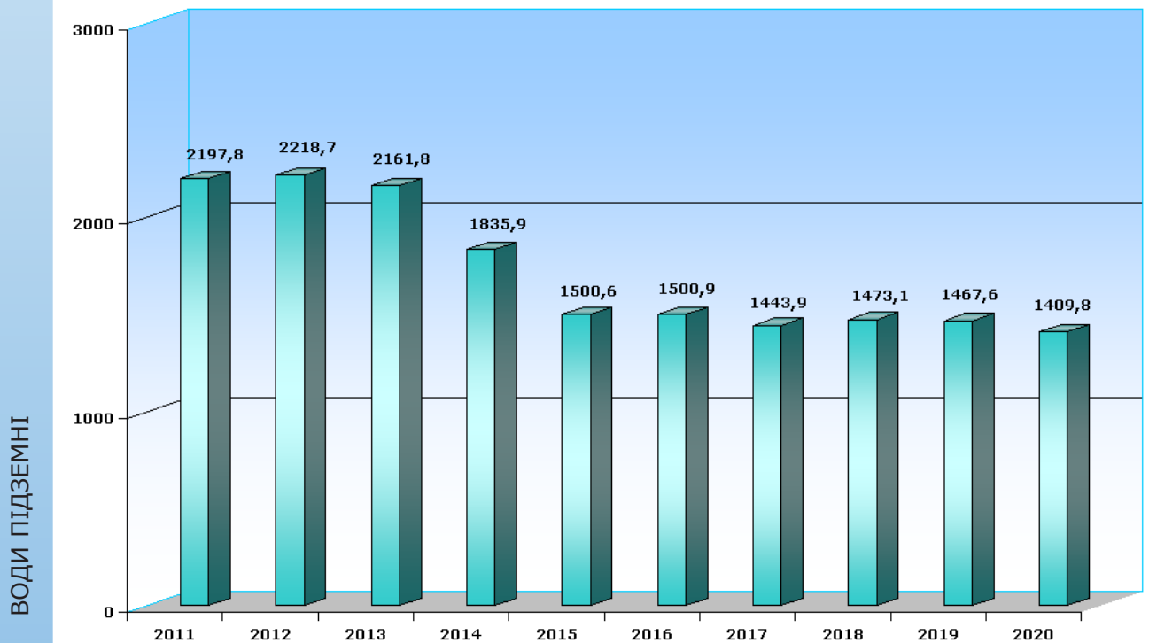
Рис. 3 - Динаміка видобутку підземних питних і технічних вод за 2011-2020 рр. (тис.м³/добу)
