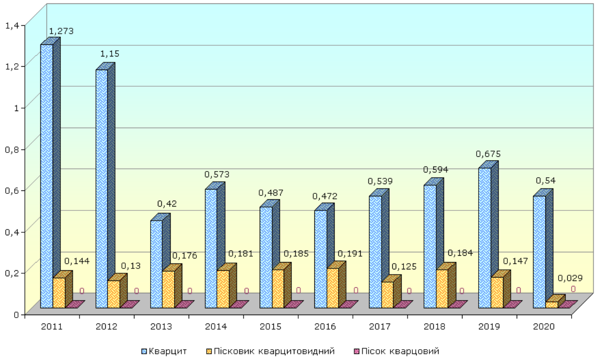
Рис. 8 - Динаміка видобутку кварциту та кварцу для вогнетривів за 2011-2020 рр., (млн.т)
