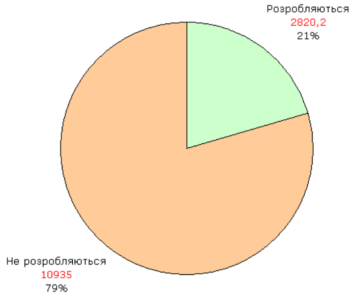
Рис. 6 - Розподіл балансових запасів графіту за ступенем промислового освоєння
