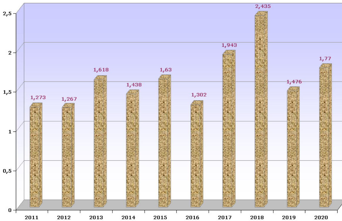
Рис. 15 - Динаміка видобутку сировини карбонатної для цукрової промисловості за 2011-2020 рр., (млн.т)
