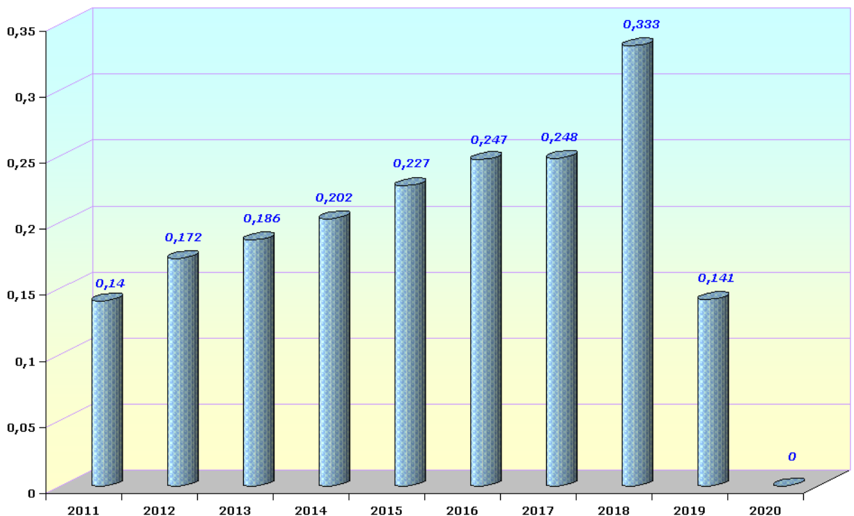
Рис. 6 - Динаміка видобутку підземних теплоенергетичних вод за 2011-2020 рр.(тис.м 3 /добу)
