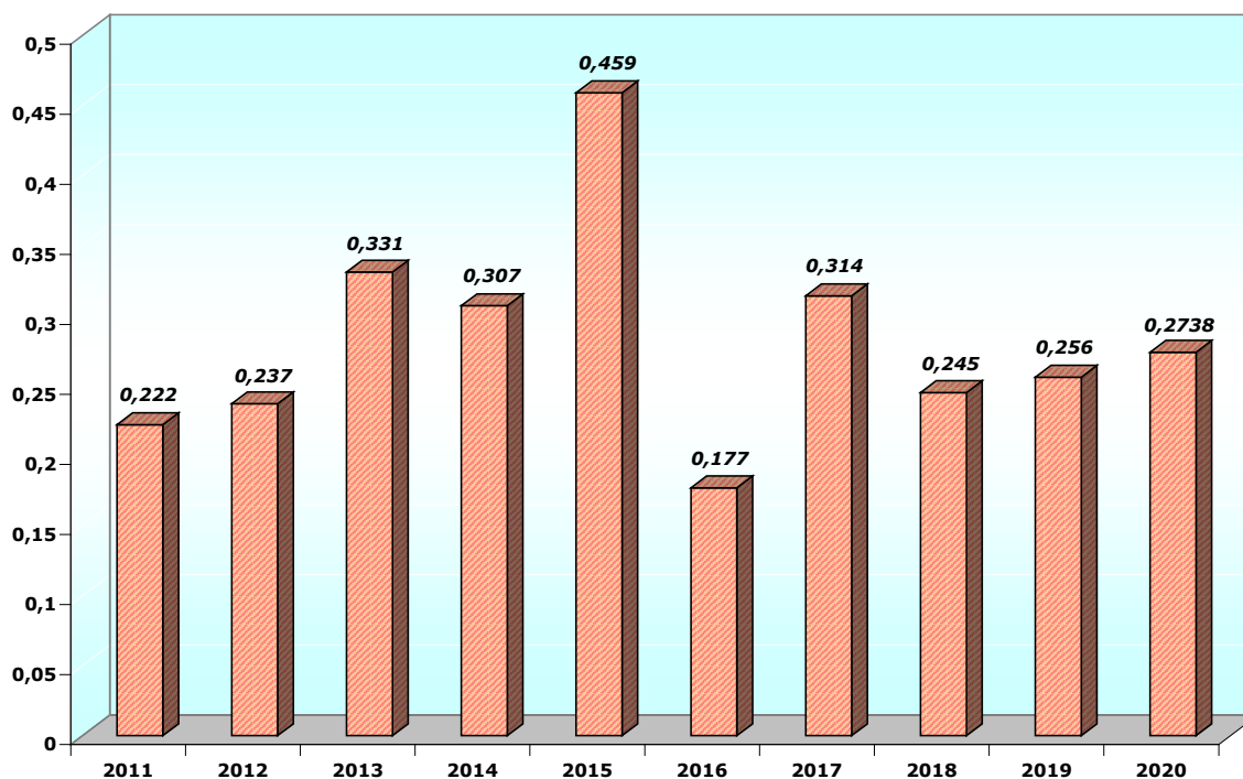
Рис. 25 - Динаміка видобутку сировини за 2011-2020 рр., (млн.м 3 )
