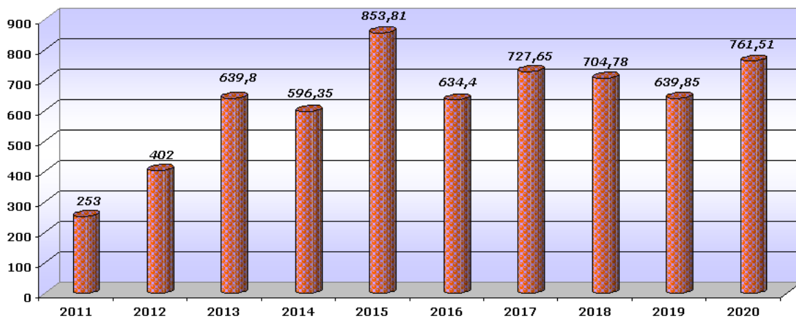
Рис. 52 - Динаміка видобутку піщано-гравійної суміші за 2011-2020 рр., (тис.м 3 )
